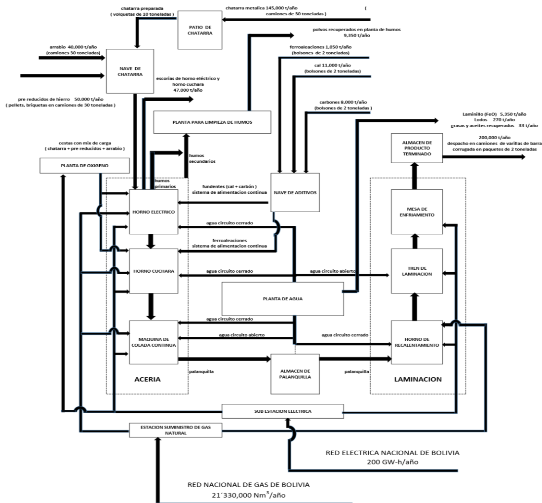
Gráfico 3: Proceso productivo de IMPORT. EXPORT. LAS LOMAS LTDA.
