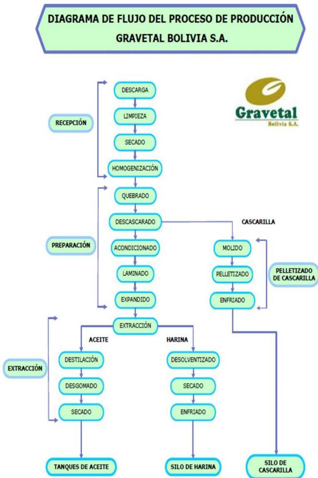
Gráfico 8: Diagrama de Flujo de Proceso
